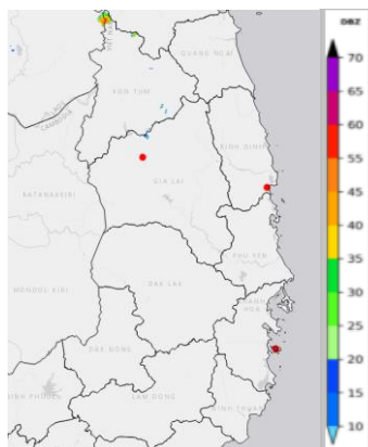
Hình 1: Ảnh ra đa thời tiết tại khu vực Tây Nguyên
